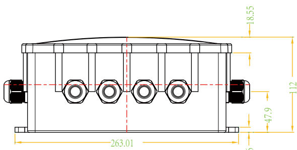
背视图
